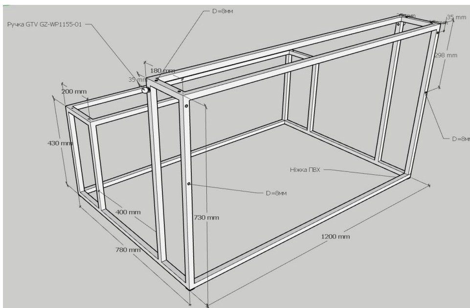
Рисунок 1 – Каркас парти з лавою
