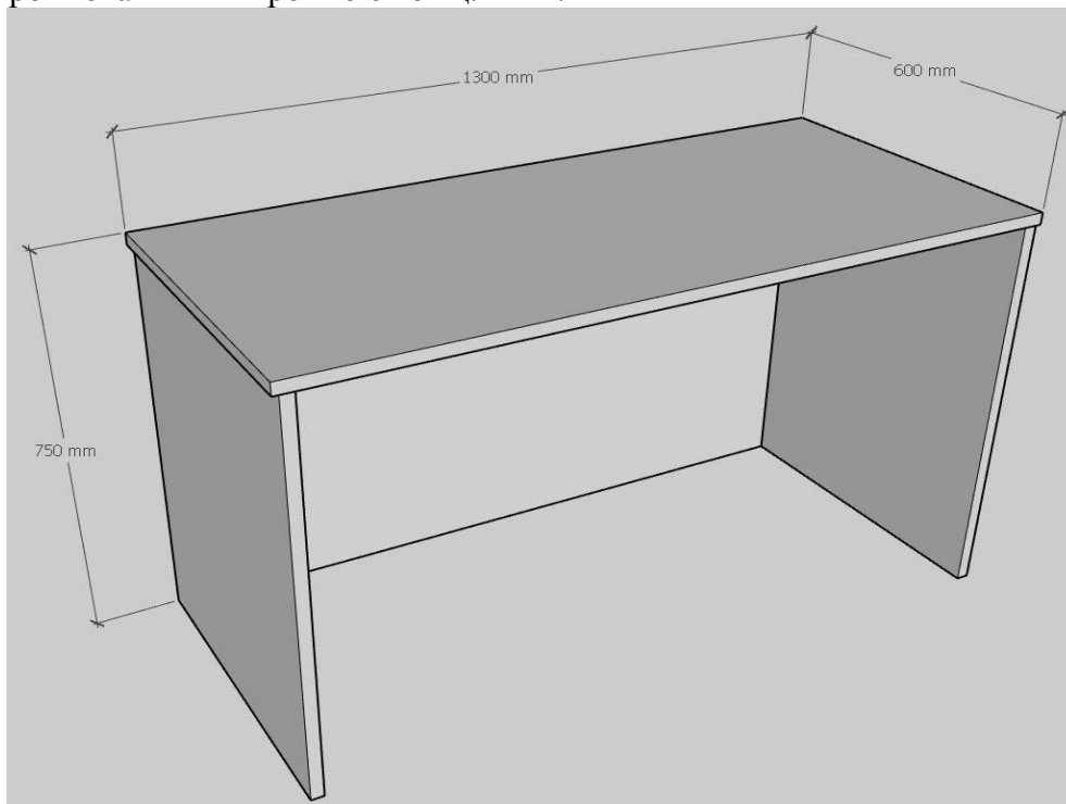
Рисунок 3 – Схематичне зображення стола викладача
