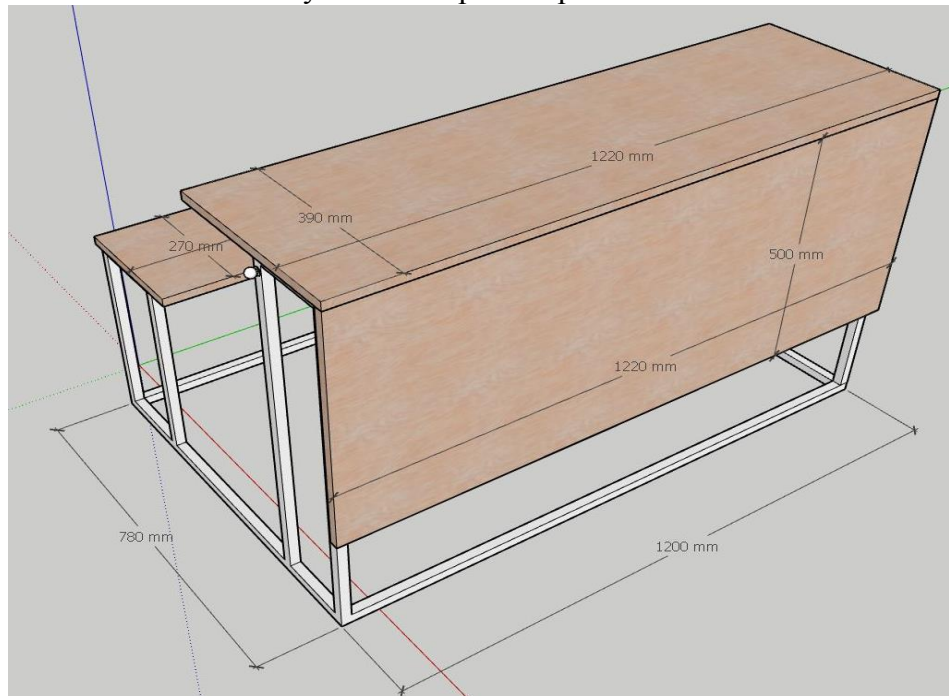
Рисунок 2 – Схематичне зображення парти з лавою
