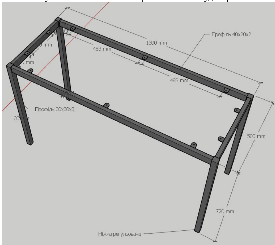
Рисунок 2 – Каркас стола аудиторного
