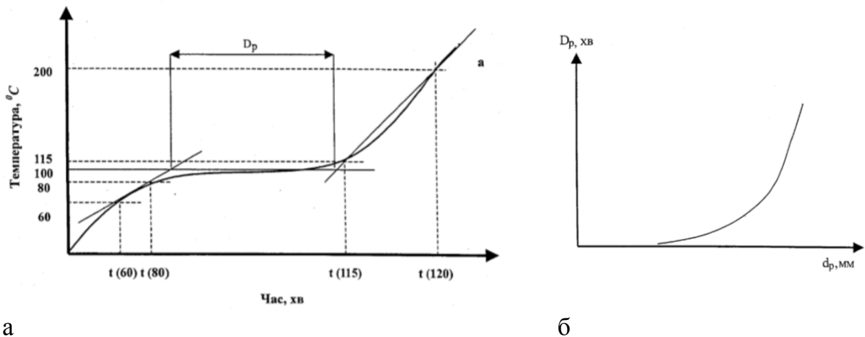
Рис. 4 Криві тривалості ізотермічної ділянки, на якій зменшується вологість покриття: а – оцінювання тривалості ізотермічної ділянки, на якій зменшується вологість покриття під час випробування; б – залежність тривалості ізотермічної ділянки, на якій зменшується вологість покриття від його товщини
