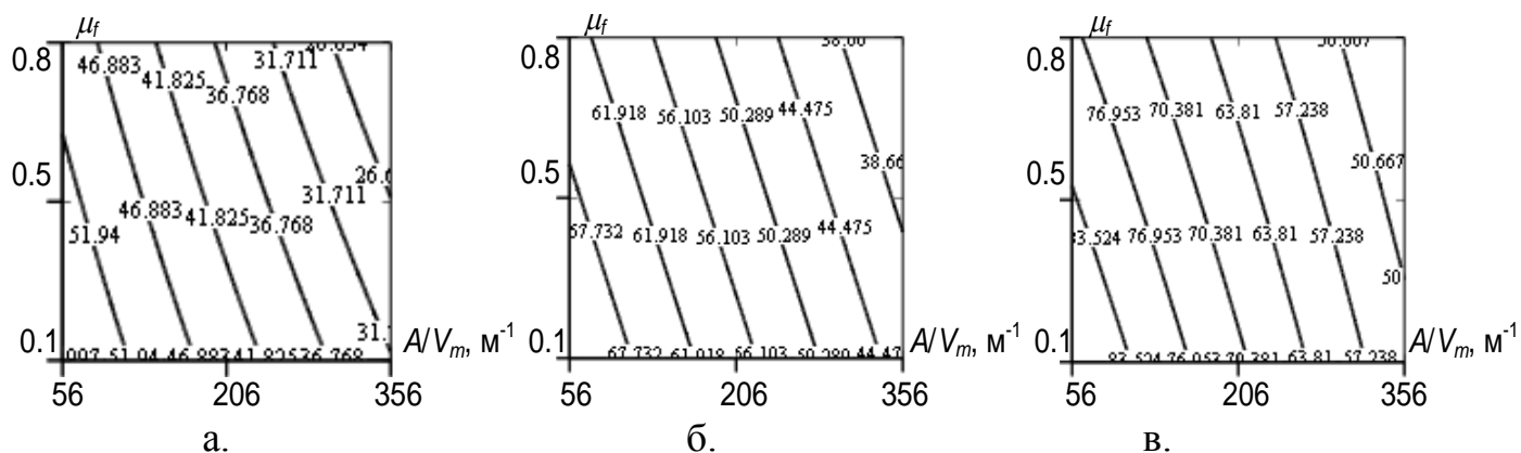
Рис. 18 Залежності час відшарування вогнезахисного мінераловатного облицювання сталевій балки від коефіцієнту перерізу та коефіцієнту навантаження для різних значень його товщини: а – 25 мм; б – 50 мм; в – 75 мм
