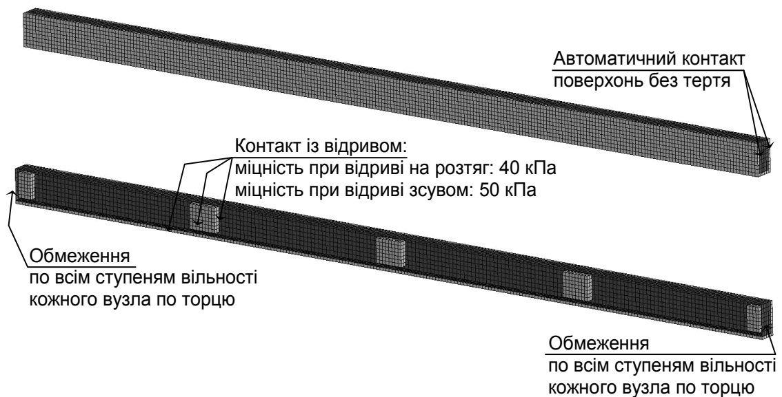
Рис. 10 Схема контактної взаємодії між елементами сталеві балки із вогнезахисним облицюванням з мінеральної вати
