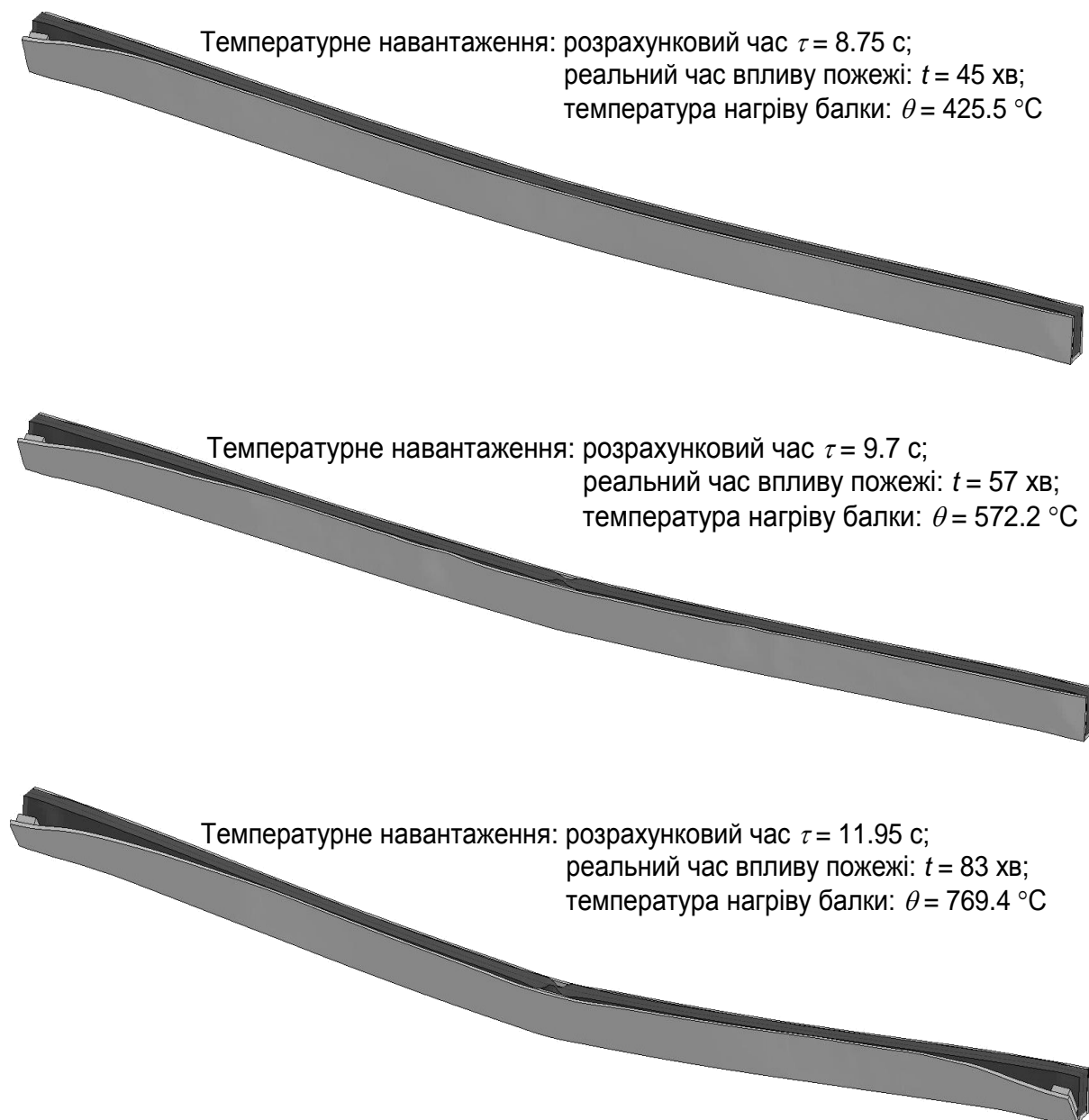
Рис. 14 Положення та геометрична форма облицювання у різні моменти часу впливу стандартного температурного режиму пожежі
